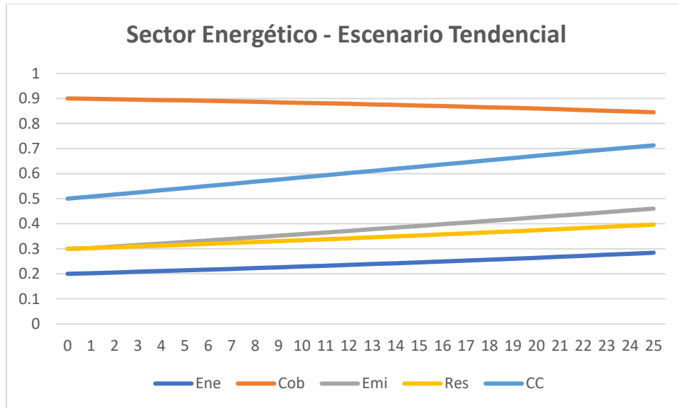
Gráfica 10 Simulación KSIM para el Sector Energético bajo el Escenario Tendencial.
